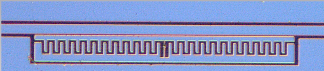
Qubit 'atom'
